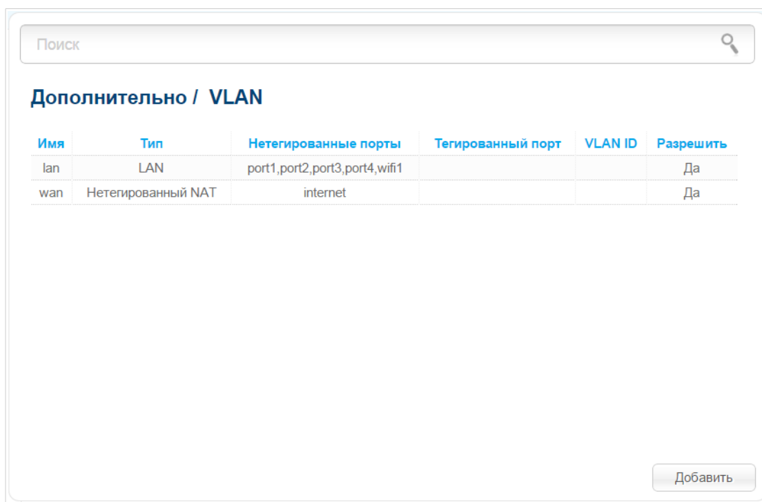
Рисунок 108. Страница Дополнительно / VLAN .
